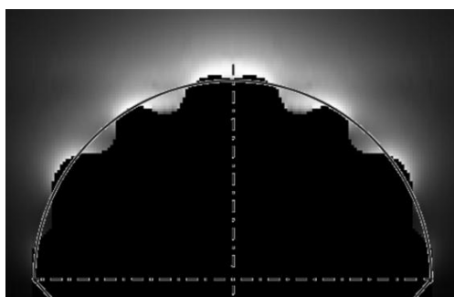
Рисунок 20 — Распределение напряжённости поля по поверхности модифицированной модели стримера. Белый — максимальное значение E
