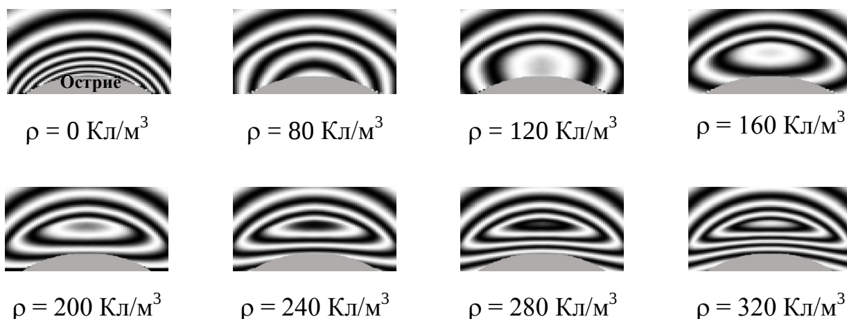
Рисунок 8 — Расчётные керрограммы. Кинограмма для набора однородных зарядов с разной объёмной плотностью \rho
