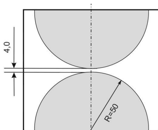
Рисунок 14 — Система сферических электродов
