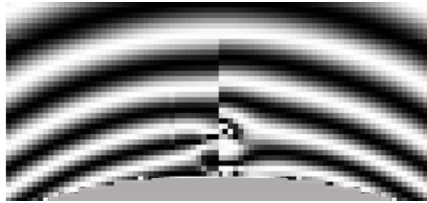
Рисунок 5 — Керрограммы. Напряжение 120 кВ, радиус кривизны острия 300 мкм. a) диэлектрический пузырёк, b) ионизированный пузырёк
