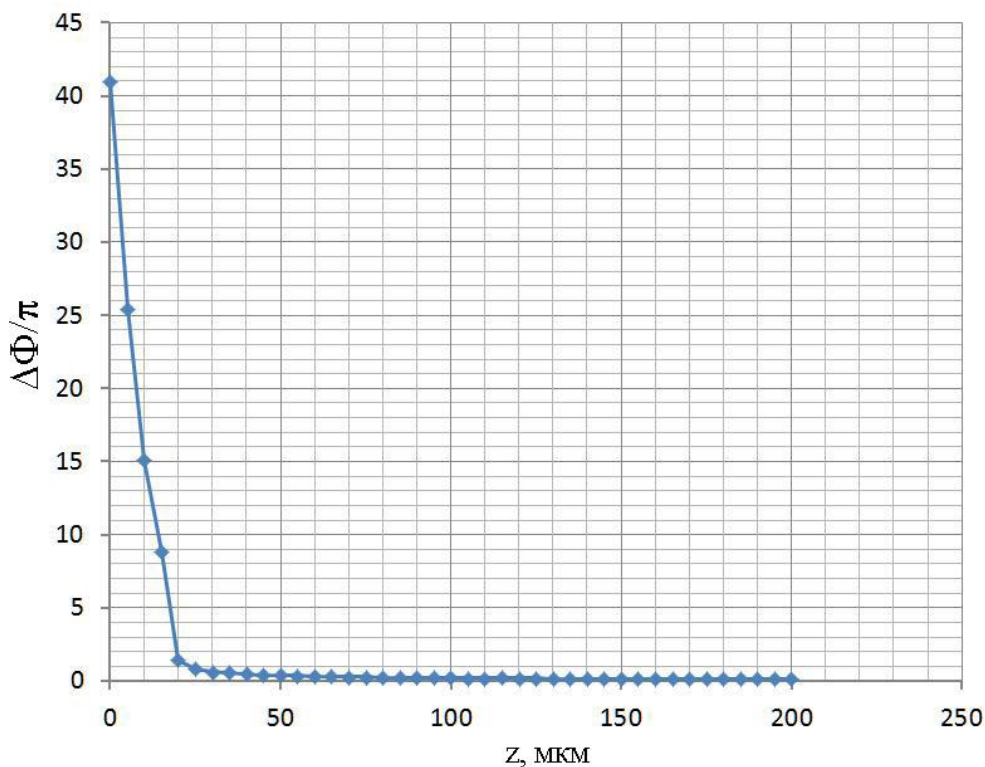
Рисунок 13 — Зависимость набег фазы \Delta\Phi/\pi от расстояния до острия по оси z при напряжении 140 кВ
