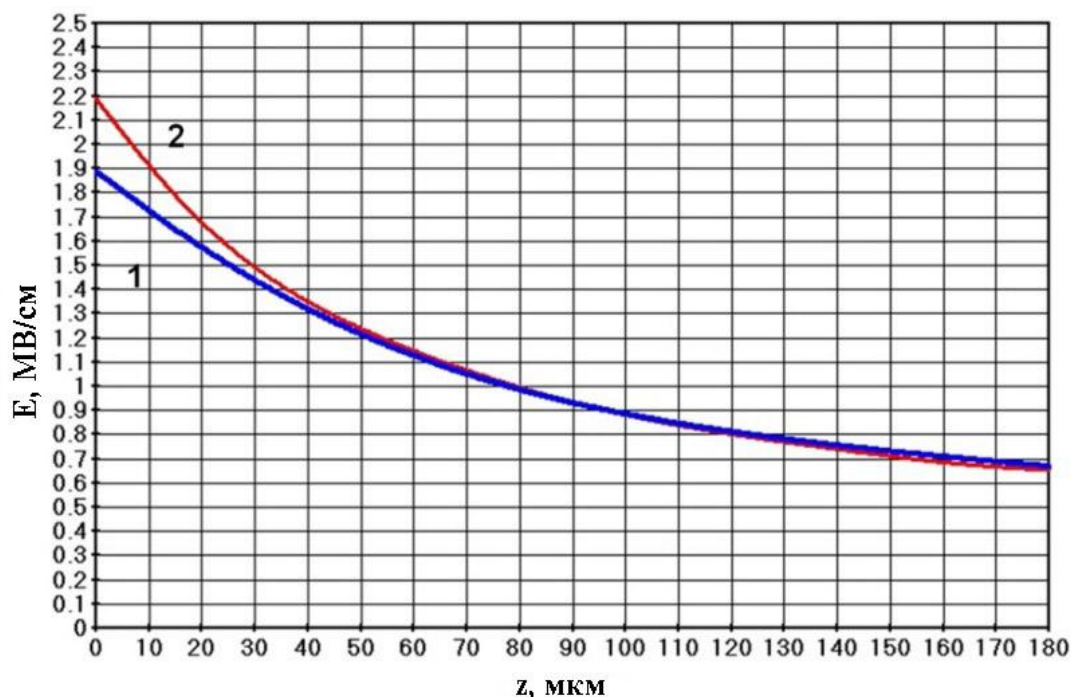
Рисунок 19 — Значения напряжённости поля на различных расстояниях от стримера по оси z : кривая 1 — \varepsilon = 80 , кривая 2 — \varepsilon = \varepsilon(E)
