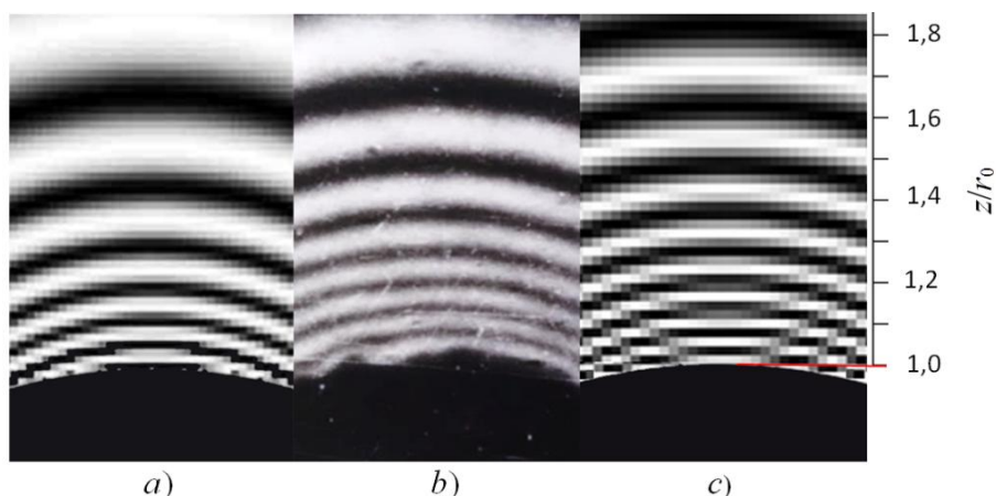
Рисунок 4 — Керрограммы: а) расчётная при B = 3,0 \times 10^{-12} \text{ м/В}^2 ; б) экспериментальная; в) расчётная, уточнённая
